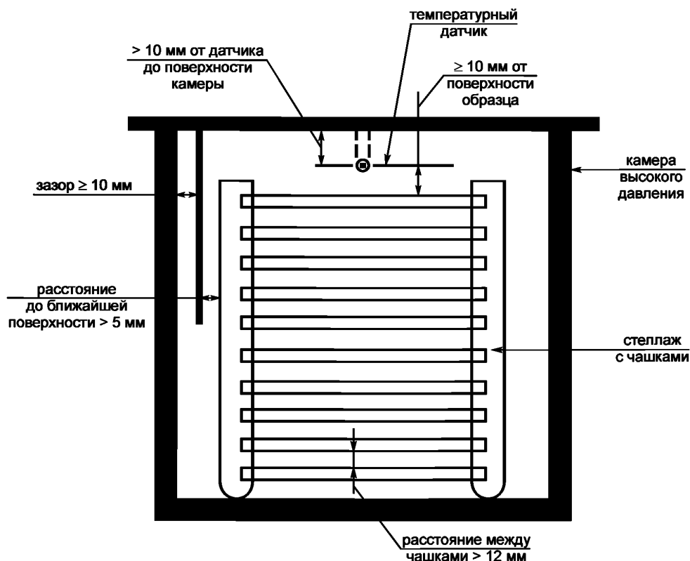
Рисунок 2 — Схема камеры высокого давления
