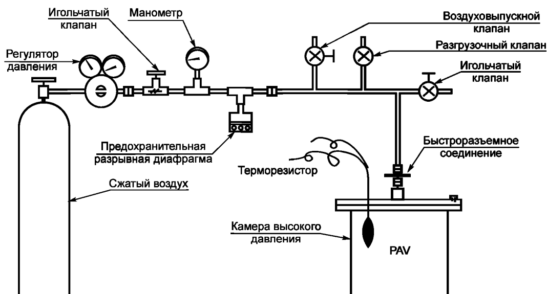
Рисунок 1 — Схема испытательного оборудования
