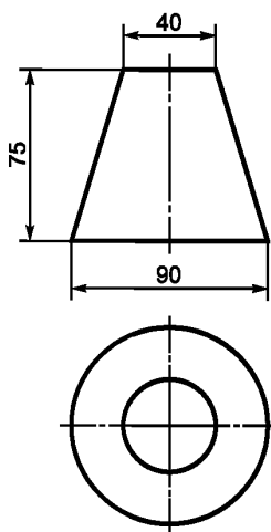
Рисунок 1 — Металлическая форма
