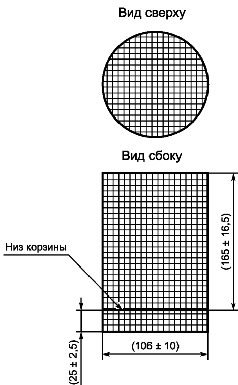
Рисунок 1 — Проволочная корзина
