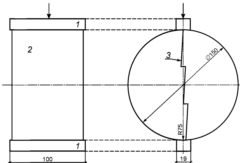
Рисунок 1 — Схема испытания на определение предела прочности при непрямом растяжении асфальтобетона
