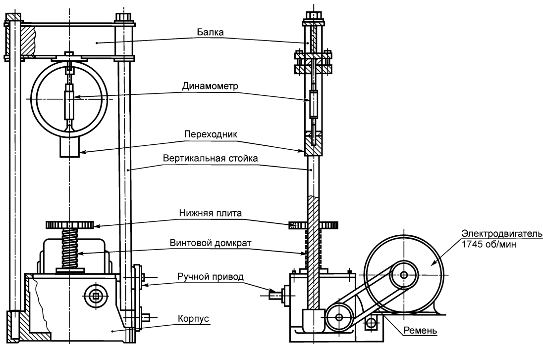
Рисунок 2 — Схема испытательной установки
