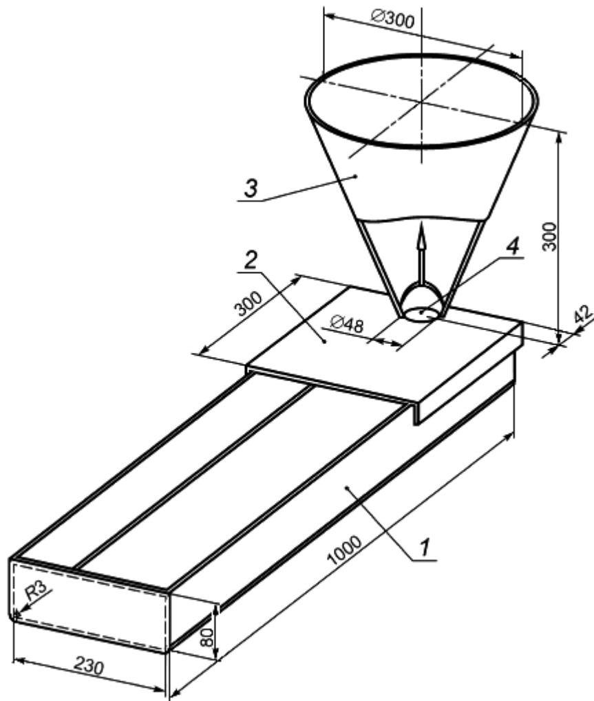
Рисунок В.3 - Стенд для испытаний ремонтных (бетонных) смесей на удобоукладываемость по текучести
