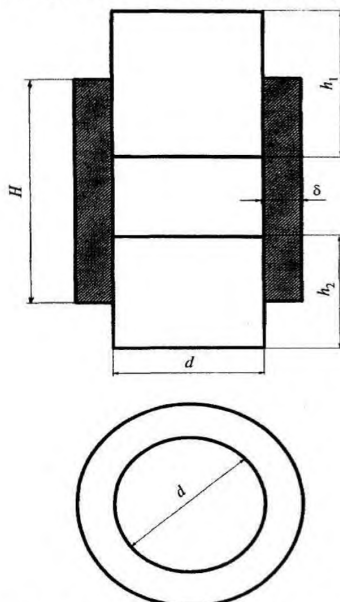
Рисунок 1 – Формы для изготовления образцов
