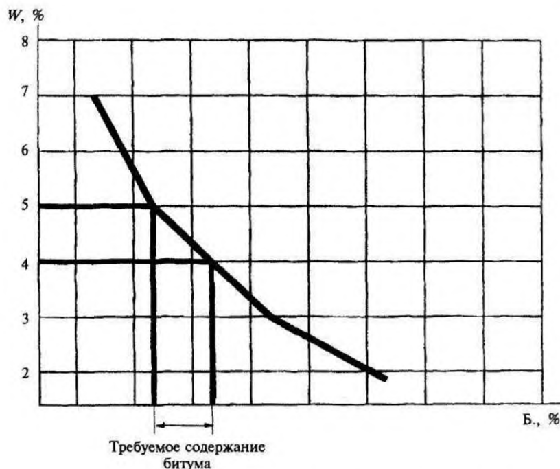
Рисунок 2 – Определение требуемого содержания битума
